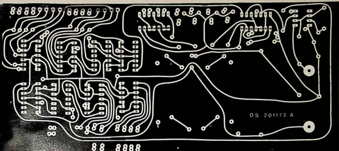
Fig. 2a. Schaakprint koperzijde.
